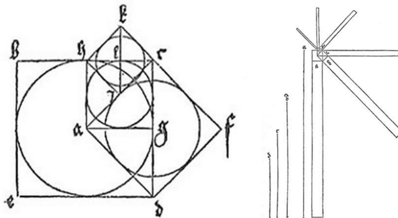
Máquina de Durero para generar líneas serpentinadas libres.
